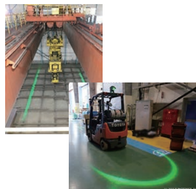
LEDライト (クレーン／フォーク移動の可視化)
